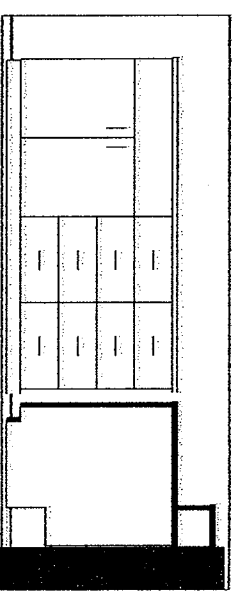
D1 ELEVATION scale: 1/2" = 1'-0"
