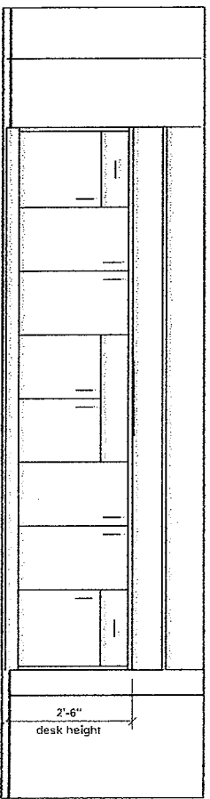
O2 ELEVATION scale: 1/2" = 1'-0"
