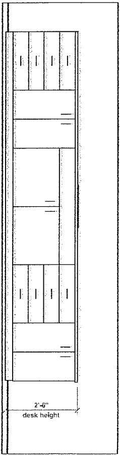
C1 ELEVATION scale: 1/2" = 1'-0"
